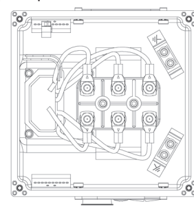
Кабельные зажимы для двигателей типоразмеров 200-280
