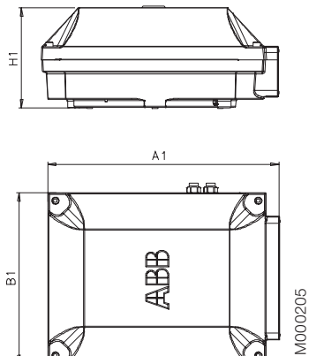
Двигатели типоразмеров 355 - 400 Монтаж сбоку Соединительная коробка 750
