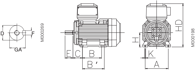
Двигатель с монтажом на лапах IM 1001, IM B3
