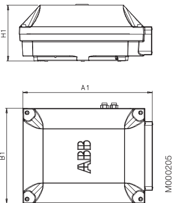
Двигатели типоразмеров 280 - 315 Монтаж сверху и сбоку Соединительные коробки 210,370
