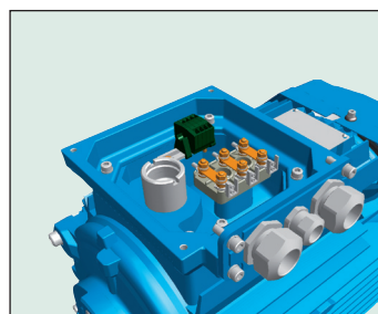
Рис. 6. Кабельные зажимы для двигателей типоразмеров 80-132
