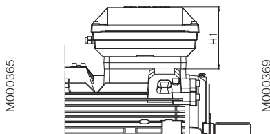
Двигатели типоразмеров 355 - 400 Монтаж сбоку Соединительная коробка 750
