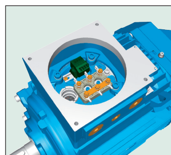
Рис. 6. Кабельные зажимы для двигателей типоразмеров 80-132
