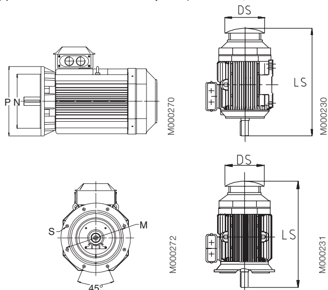
Защитный кожух, код модификации 005
