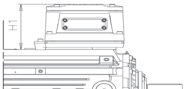
Двигатели типоразмеров 355 - 400 Монтаж сверху Соединительная коробка 750 + переходник
