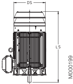
Двигатель с защитным кожухом
