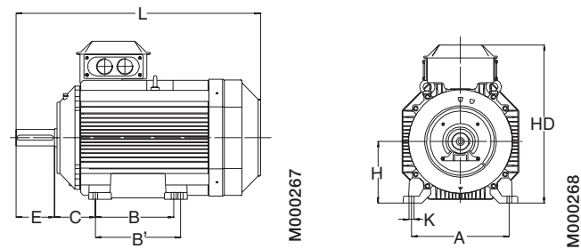
Двигатель с монтажом на лапах IM 1001, IM B3
