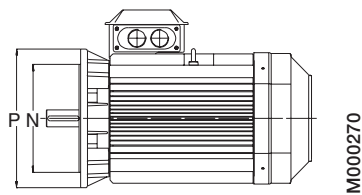
Двигатель с монтажом на фланце IM 3001, IM B5
