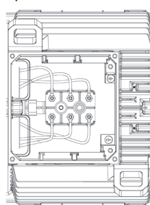
Кабельные зажимы для двигателей типоразмеров 160-180
