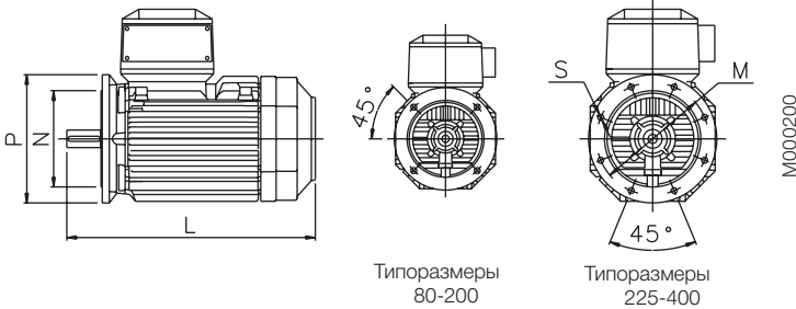
Двигатель с монтажом на фланце IM 3001, IM B5
