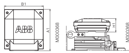
Двигатели типоразмеров 280 - 315 Монтаж сверху и сбоку Соединительные коробки 210,370
