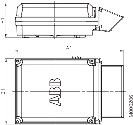
Двигатели типоразмеров 355 - 400 Монтаж сверху Соединительная коробка 750 + переходник
