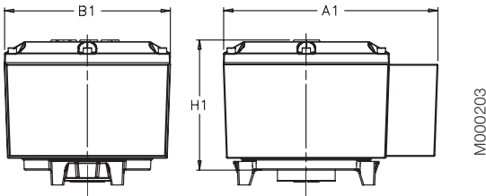
Двигатели типоразмеров 280-315
