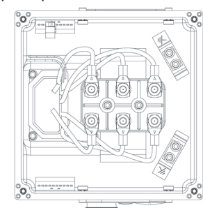
Кабельные зажимы для двигателей типоразмеров 200-280
