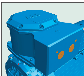
Рис. 5. Соединительная коробка для двигателей типоразмеров 355-400
