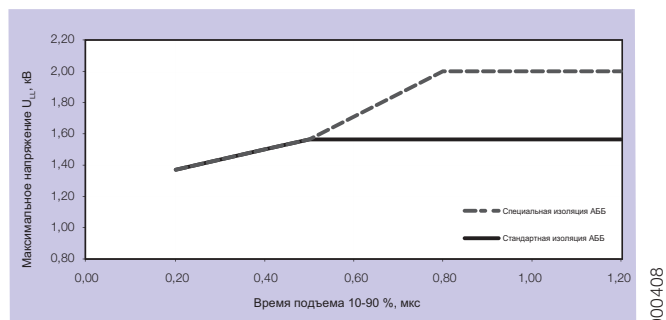
Рис. 1. Допустимые пики линейных напряжений на клеммах двигателя в зависимости от времени нарастания импульсов.
