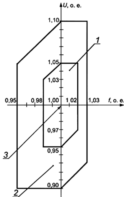
Рис. 2.7.1. Допустимые отклонения параметров сети
